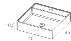
lav. pousar_ CALAMA cerâmico
